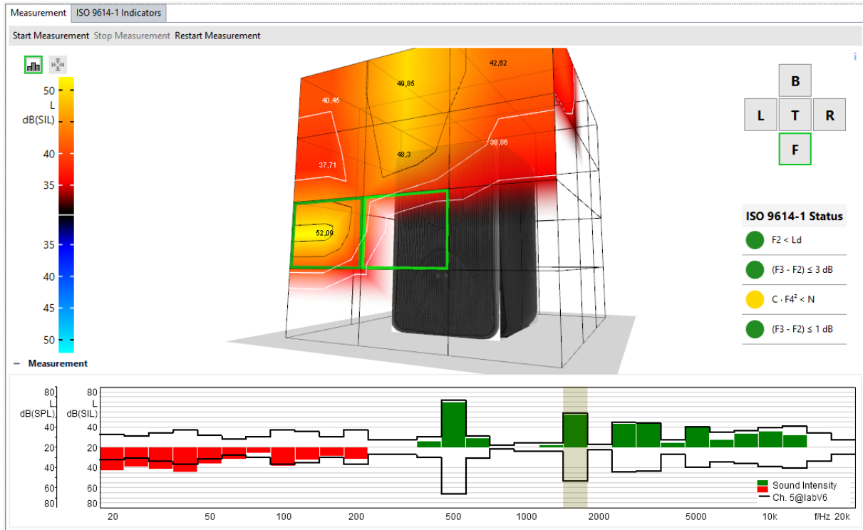
Schalleistungsmessung in ArtemiS SUITE 10.0.
